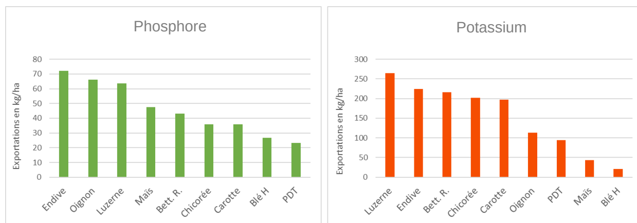
Figure 1. Exportation de phosphore et potassium pour différentes cultures pour un rendement moyen (le rendement moyen est calculé parmi les producteurs mobilisés dans l'étude, Agro-Transfert, projets VivLéBio)
