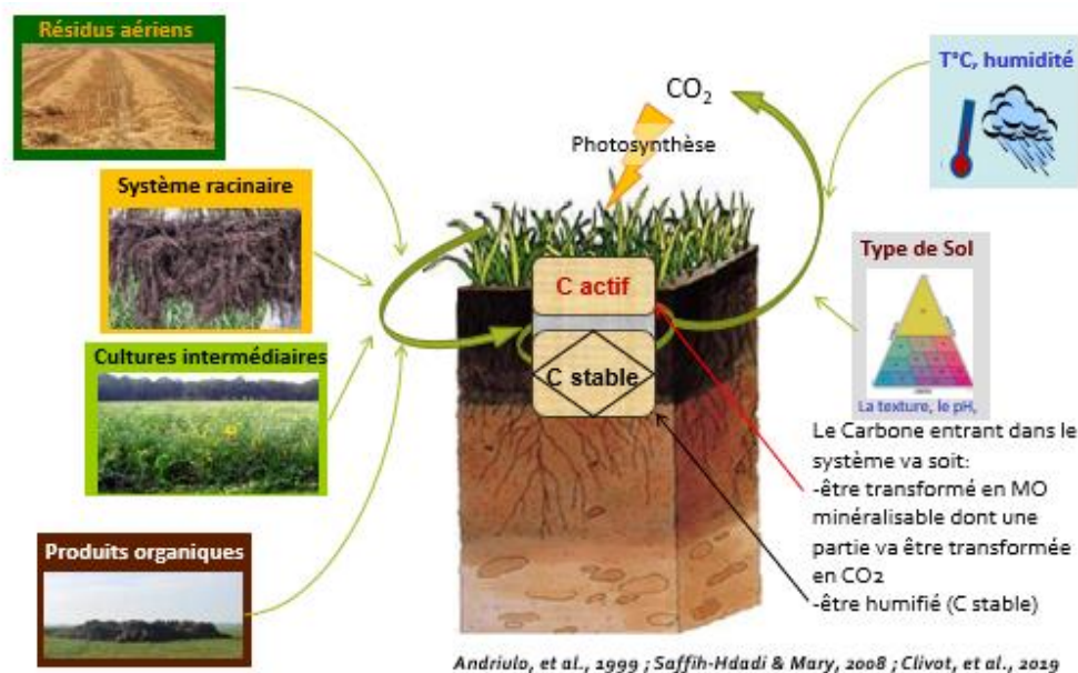
Figure 3. Flux de carbone dans le sol
