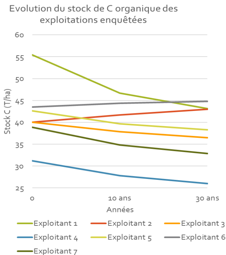
Figure 4. Simulation de l'évolution du stock de carbone organique pendant 30 ans dans les exploitations enquêtées
