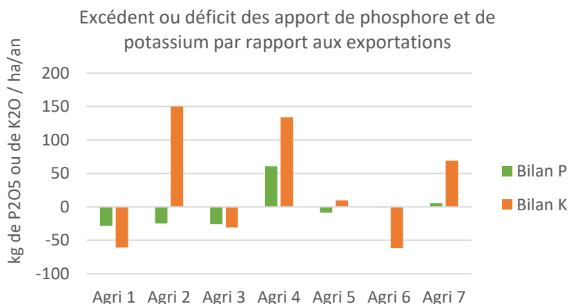
Figure 2. Bilan en phosphore et potassium de différentes exploitations
