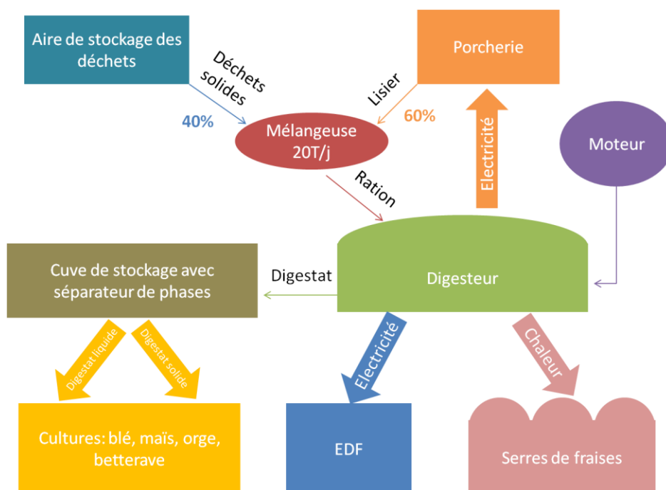
Schéma illustrant le fonctionnement du système de Sébastien Manscourt
